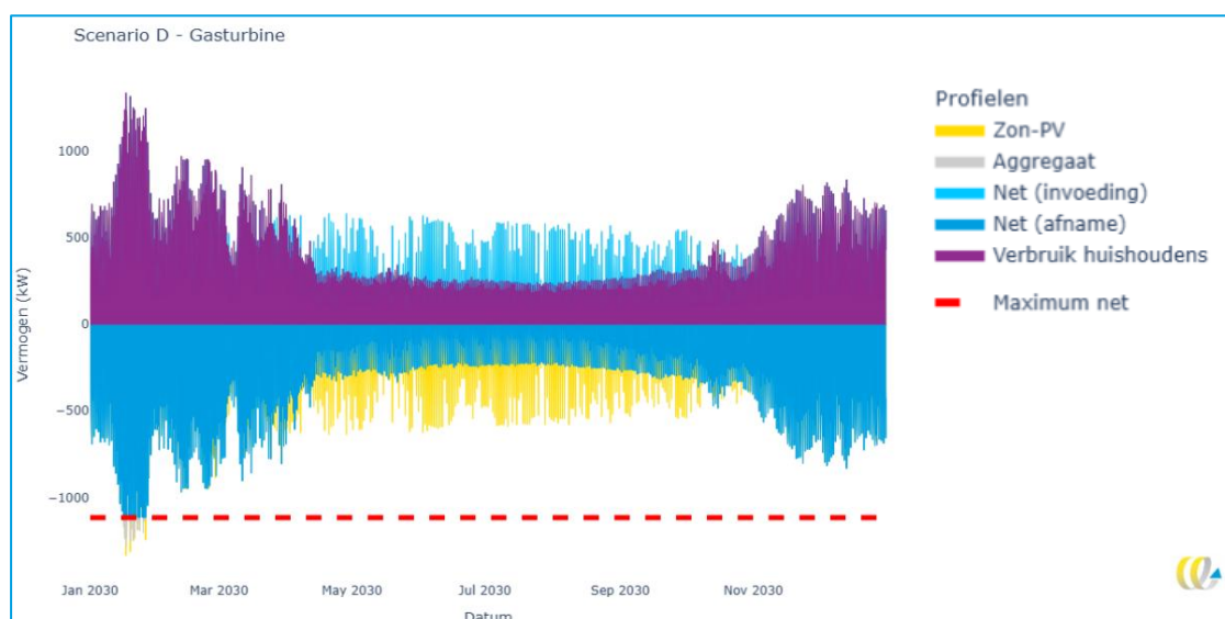
Figuur 20 – Jaarlijks energievraag en -aanbod voorbeeldwijk: Scenario D 'Gasturbine'
